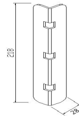
3、连接件样板
